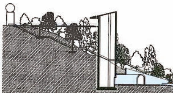
Fig. 1 - Corte longitudinal - desenho extraído do projeto.
